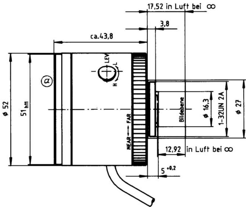
Cinegon 1,8/4,8 in mot. Blendenregler (VS)
